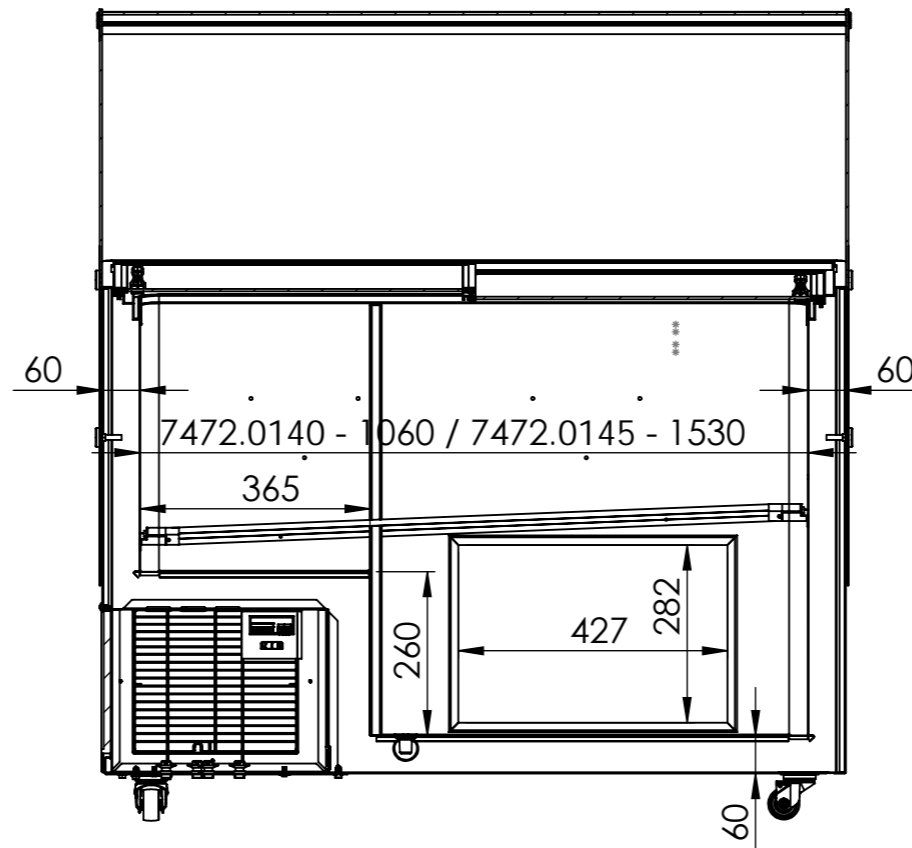
SECTION B-B SCALE 1 : 12
